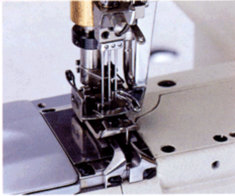
調節式布誘導器、活動壓腳舌。 Adjusting fabric guide, and adjustable presser foot.
